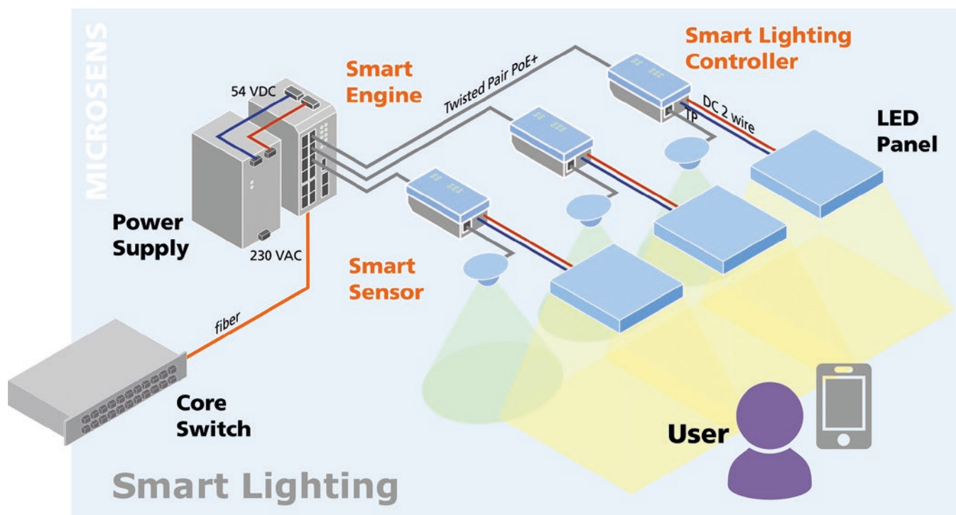
Abb. 3: Die innovative MICROSENS Smart Lighting-Lösung. LED-Leuchten werden durch PoE+ über eine normkonforme Verkabelung nach DIN EN 50173-6 mit Strom versorgt. Sensoren in Leuchtennähe liefern die Daten zu Helligkeit, Temperatur und Anwesenheit von Personen im Raum. Die Smart Director App auf den Micro-Switches regelt die Beleuchtung nach den Bedürfnissen der Anwender.
