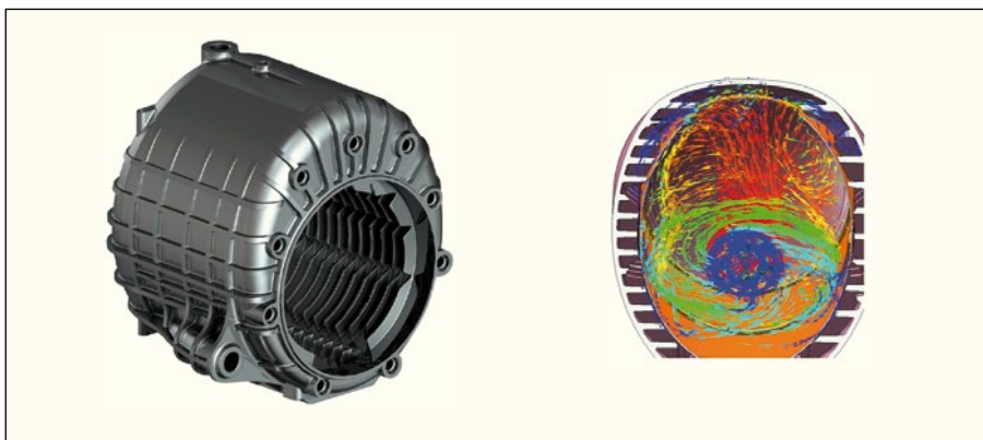
Abb.2: Primär-Wärmetauscher in AL/SI-Legierung als Monoblock in einem Stück gegossen.
