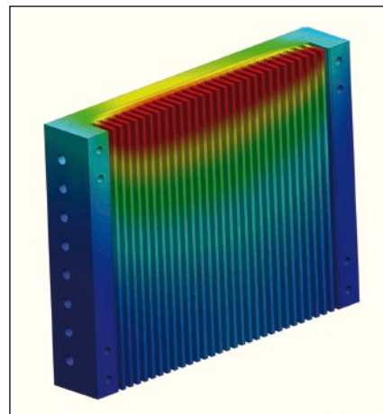
Abb.4: Wärmeübertragung im Carbon-Wärmetauscher
