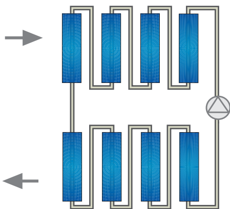
Abb. 1 Reihenschaltung der Wärmeübertragerstufen
