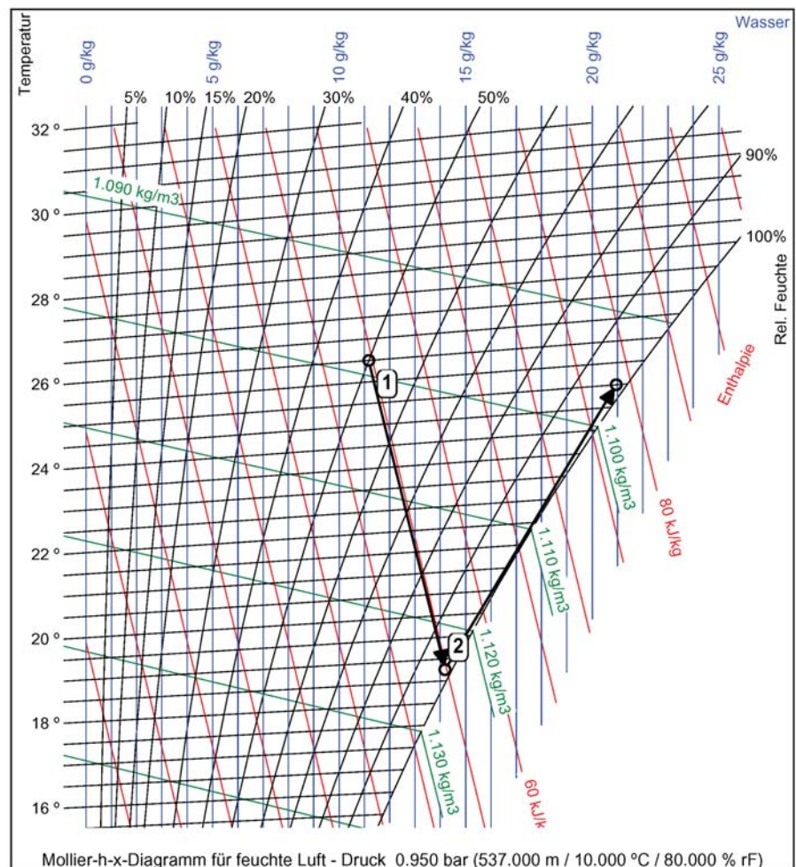
Abb. 4 Idealisierte Zustandsänderung im indirekten Verdunstungsbefeuchter
