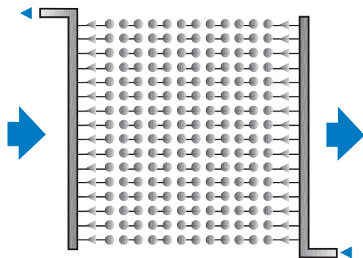
Abb. 5 Kreuz-/Gegenstromschaltung von Rippenrohrwärmeübertragern
