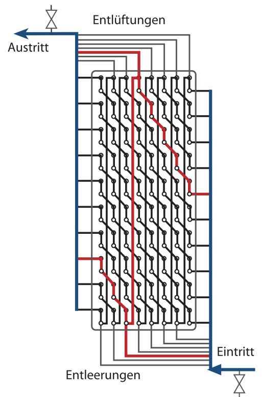
Abb. 6 Fallende Gegensinnverrohrung mit Entlüftung und Entleerung [10]
