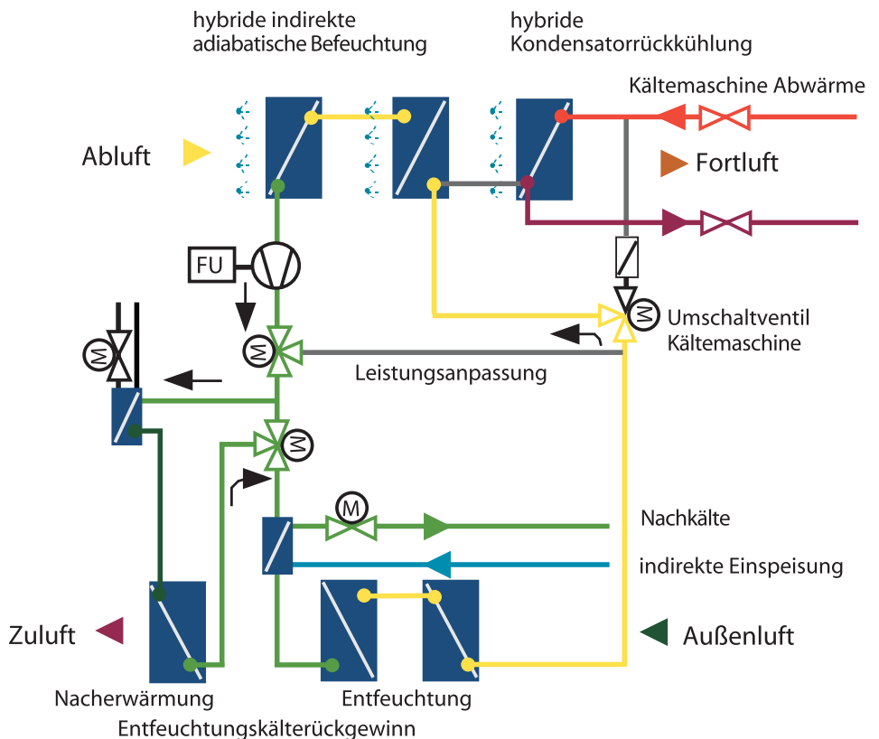
Abb. 8 Erweiterte Sekundärfunktionen im Sommerbetrieb
