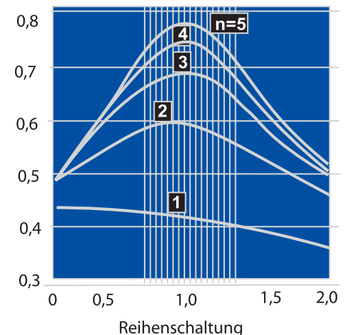
Abb. 2 Temperaturaustauschgrad als Funktion des Wärmestromkapazitätsverhältnisses bei k \times A / W_W = \text{const.} [4]
