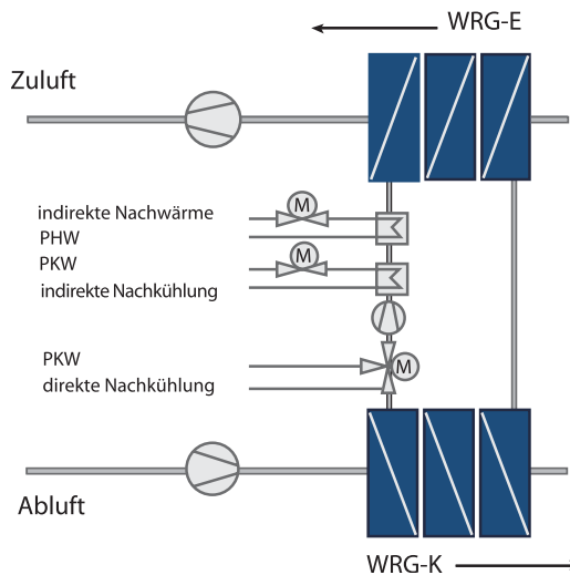
Abb. 7 Wärmeeinspeisung bzw. Wärmeauskopplung in das Hochleistungs-KV-System
