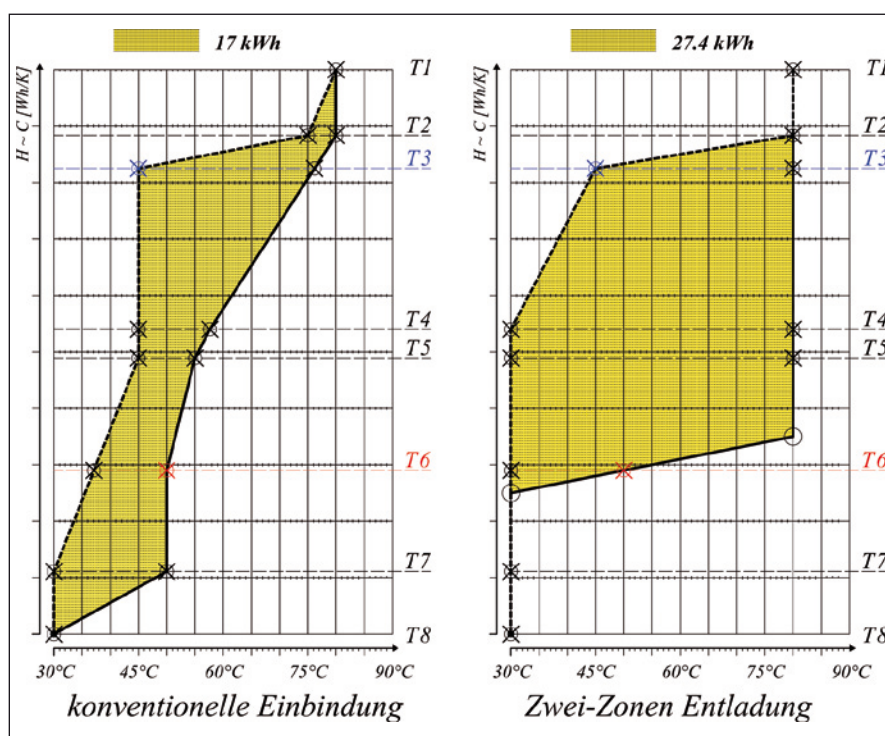
Abb. 9: Effektive spezifische Wärmemenge eines real vermessenen Pufferspeichers
