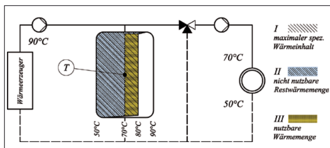
Abb. 5: Effektive spezifische Wärmemenge eines ideal durchmischten Speichers
