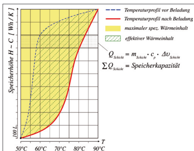
Abb.3: Maximaler spezifischer Wärmeinhalt in Abhängigkeit vom Temperaturprofil im Speicher und der Verbraucher-Rücklauftemperatur
