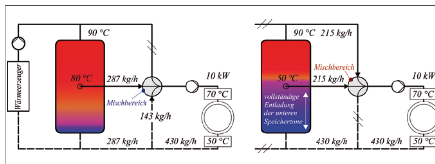
Abb. 8: Zwei-Zonen-Entladung
