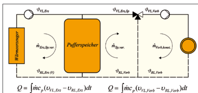
Abb.2: Be- und Entladung eines Heizwasserspeichers
