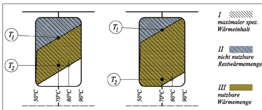
Abb. 7: Effektive spezifische Wärmemenge eines linear geschichteten Speichers
