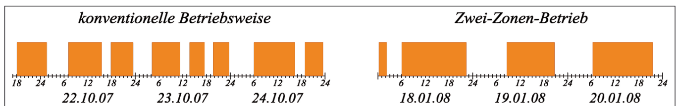
Abb. 1: Taktverhalten des BHKWs im konventionellen- bzw. Zwei-Zonen-Betrieb
