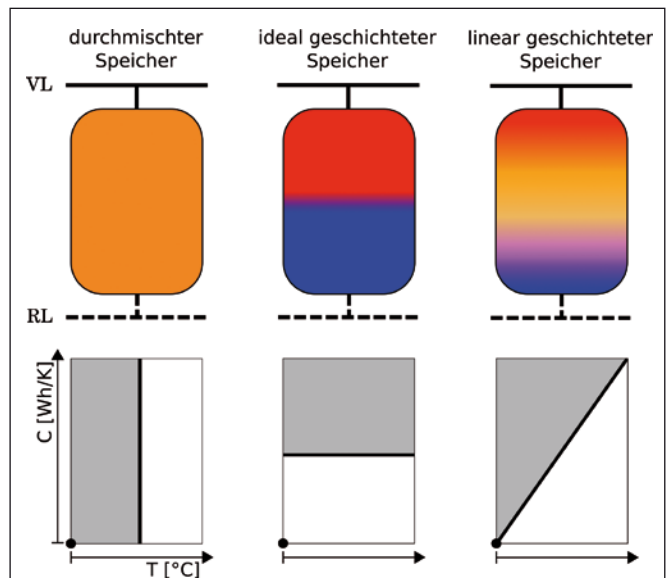
Abb. 4: Idealisierte Speichermodelle samt Temperaturverteilung
