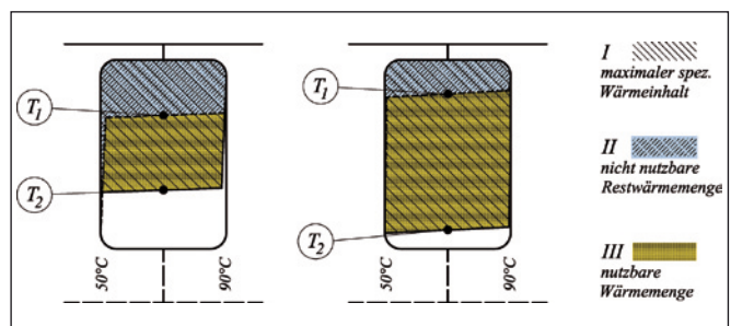
Abb. 6: Effektive spezifische Wärmemenge eines ideal geschichteten Speichers
